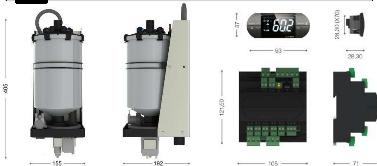
UMIDIFICATORE ES-OEM-CCU
